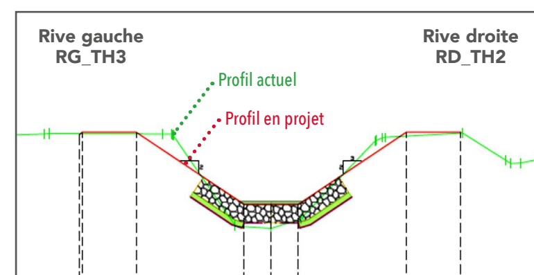
Profil illustrant le principe de remodelage et de renforcement des berges du Piésan (Source : Présentation de la réunion publique du 5 juin 2025)
