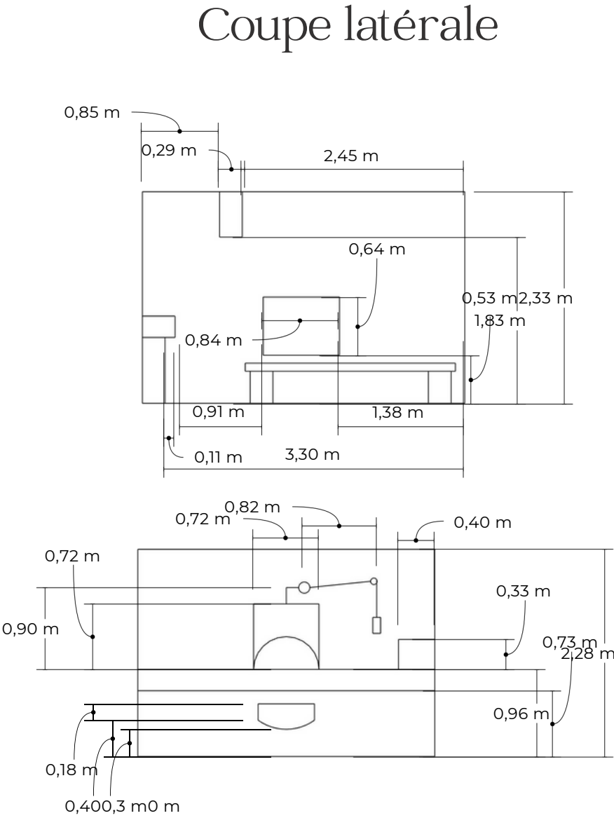
Coupe
